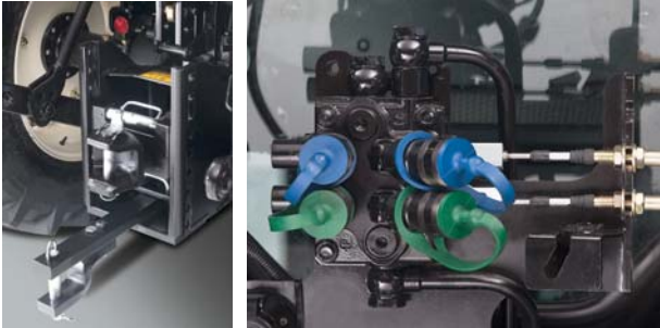
Farklı ekipman kullanımına imkanı sağlayan sabit ve kayarlı çeki sistemi 4 adet damper çıkışı
